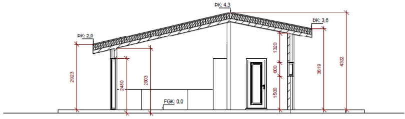
Sneiðmynd BB
