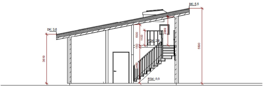
Sneiðmynd AA
